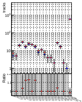
N of reco track vs. \chi^2 —•— DQM CKF TTbase —•— DQM CKF TT_retrainOldFiles125_v2_prelimWPM_epoch3
