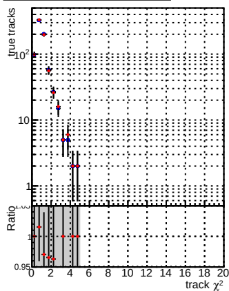
N of reco track vs. \chi^2 —•— DQM CKF TTbase —•— DQM CKF TT_retrainOldFiles125_v2_prelimWPM_epoch3
