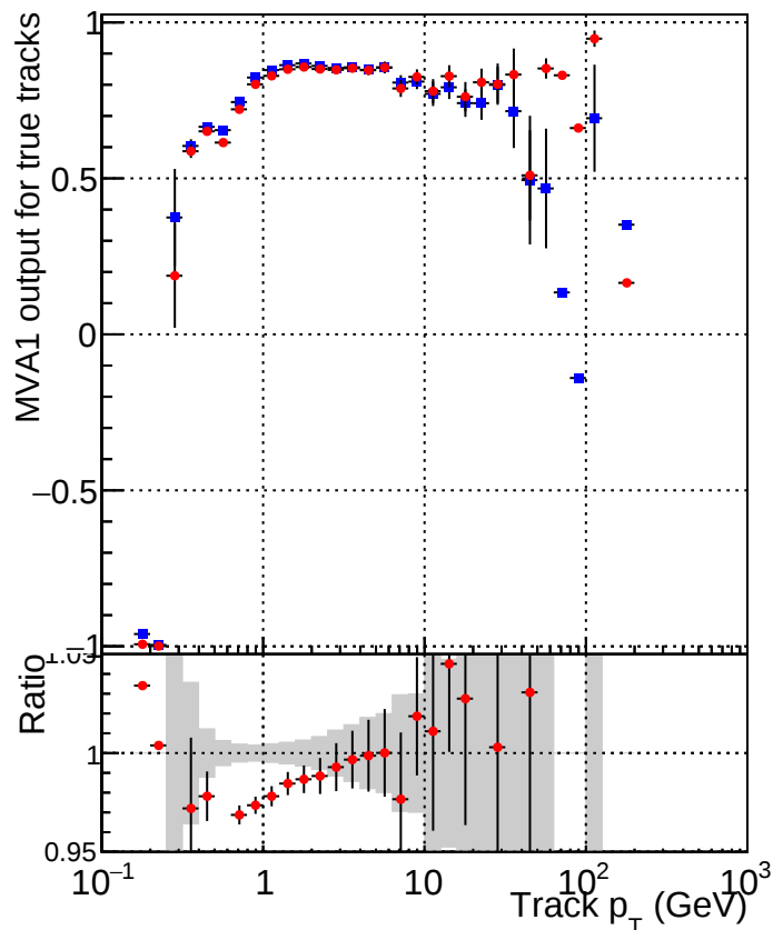
■ DQM_CKF_TTbase ◆ DQM_CKF_TT_retrainOldFiles125_v2_prelimWPM_epoch3
