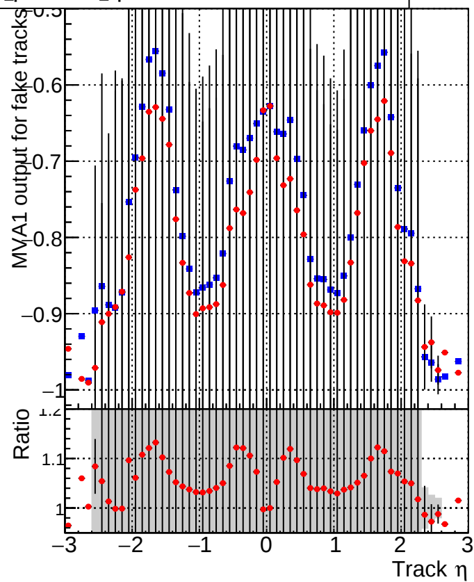
■ DQM_CKF_TTbase ◆ DQM_CKF_TT_retrainOldFiles125_v2_prelimWPM_epoch3
