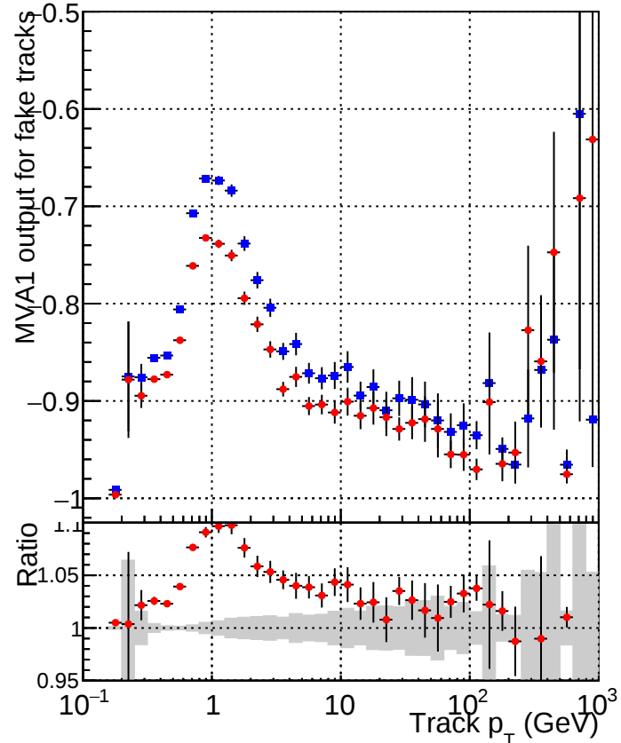
■ DQM_CKF_TTbase ◆ DQM_CKF_TT_retrainOldFiles125_v2_prelimWPM_epoch3
