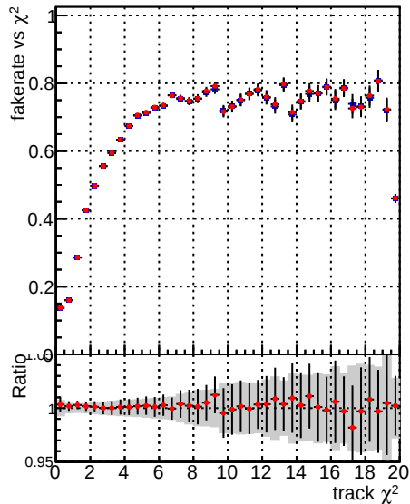
Fake rate vs. \chi^2 Legend: —•— DQM CKF TTbase —•— DQM CKF TT_retrainOldFiles125_v2_prelimWPM_epoch3
