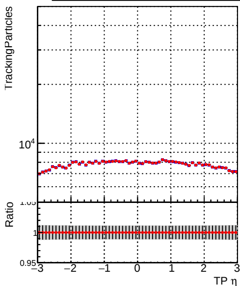
■ DQM_CKF_TTbase ● DQM_CKF_TT_retrainOldFiles125_v2_prelimWPM_epoch3
