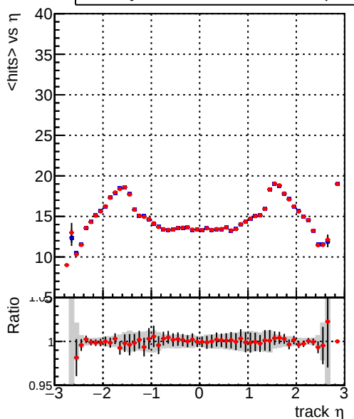
— DQM_CKF_TTbase — DQM_CKF_TT_retrainOldFiles125_v2_prelimWPM_epoch3
