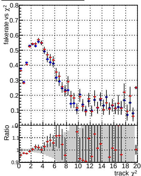
Fake rate vs. —•— DQM CKF TTbase —•— DQM CKF TT_retrainOldFiles125_v2_prelinWPM_epoch3
