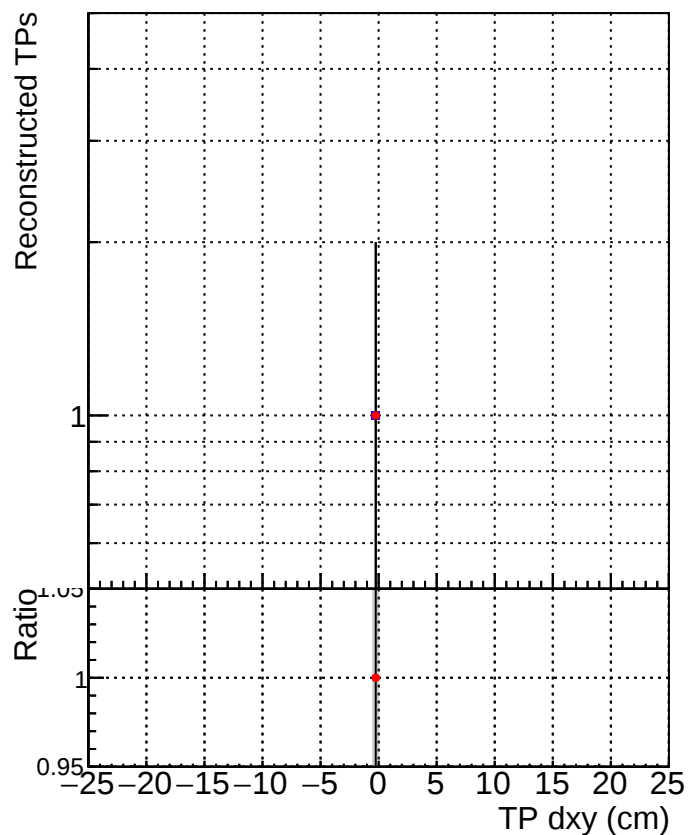
DQM_CKF_TTbase DQM_CKF_TT_retrainOldFiles125_v2_prelimWPM_epoch2
