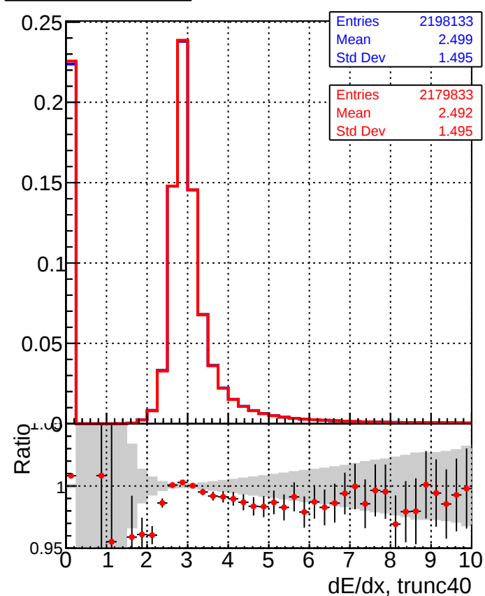
DQM_CKF_TTbase DQM_CKF_TT_retrainOldFiles125_v2_prelimWPM_epoch2
