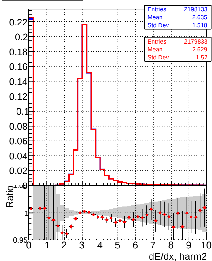
DQM_CKF_TTbase DQM_CKF_TT_retrainOldFiles125_v2_prelimWPM_epoch2
