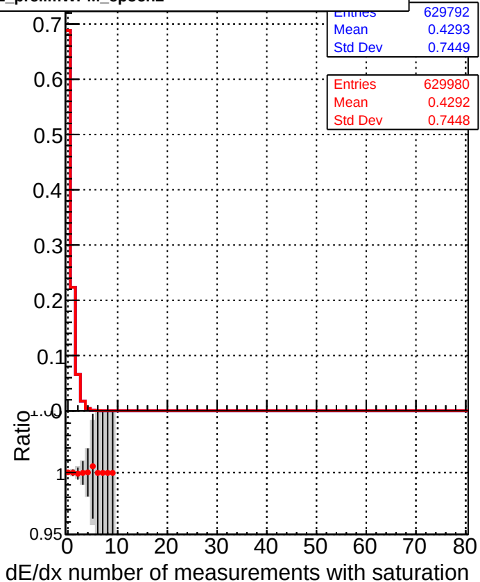
DQM_CKF_TTbase DQM_CKF_TT_retrainOldFiles125_v2_prelimWPM_epoch2
