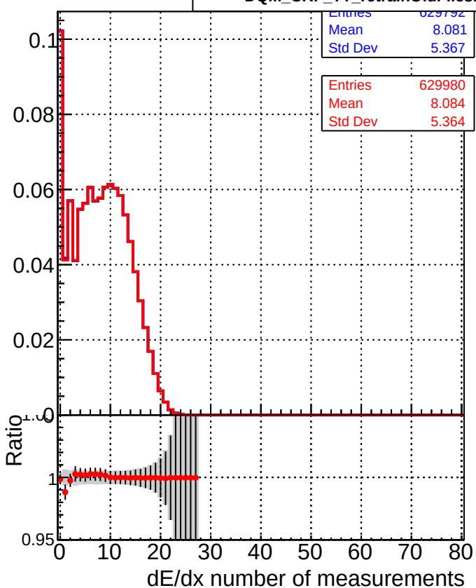
DQM_CKF_TTbase DQM_CKF_TT_retrainOldFiles125_v2_prelimWPM_epoch2
