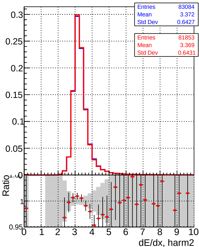
■ DQM_CKF_TTbase ● DQM_CKF_TT_retrainOldFiles125_v2_prelimWPM_epoch2
