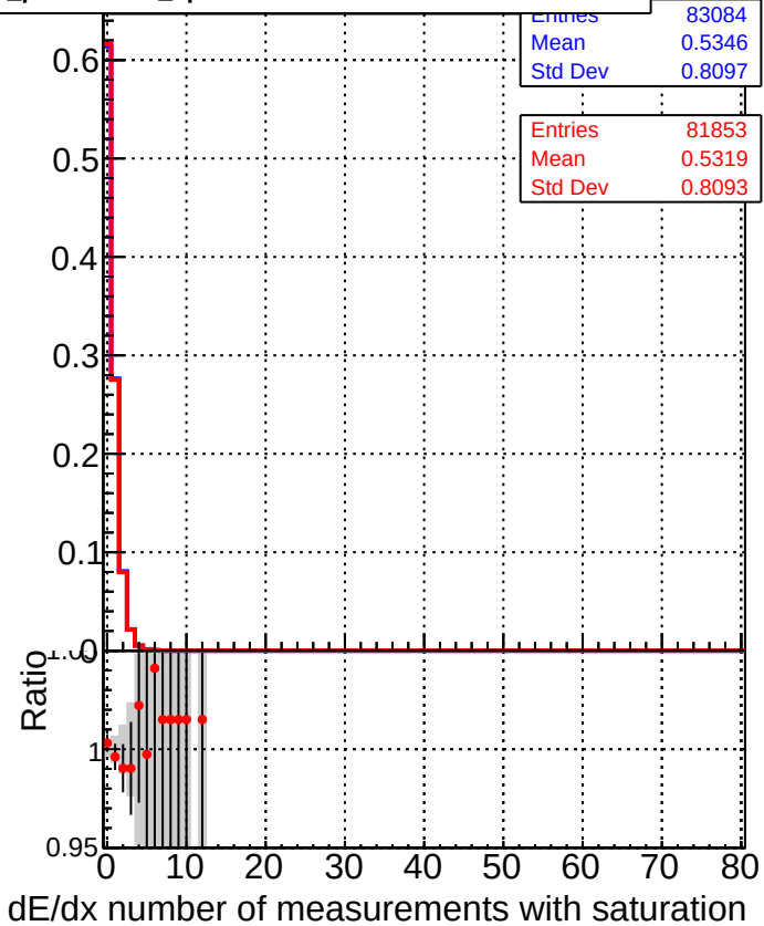
■ DQM_CKF_TTbase ● DQM_CKF_TT_retrainOldFiles125_v2_prelimWPM_epoch2
