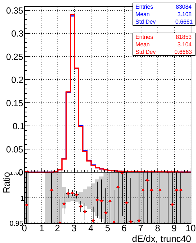
■ DQM_CKF_TTbase ● DQM_CKF_TT_retrainOldFiles125_v2_prelimWPM_epoch2
