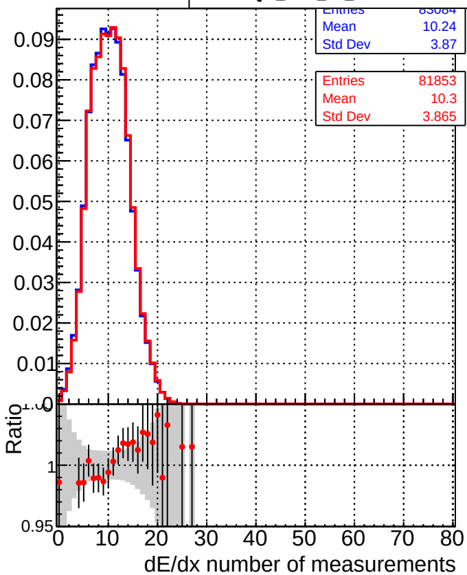
■ DQM_CKF_TTbase ● DQM_CKF_TT_retrainOldFiles125_v2_prelimWPM_epoch2
