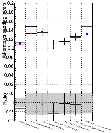
Fake rate vs. DQM CKF TTbase DQM CKF TT_retrainOldFiles125_v2_prelimWPM_epoch2
