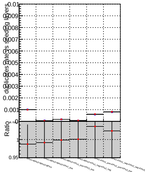
—●— DQM CKF TTbase —●— DQM CKF TT_retrainOldFiles125_v2_prelimWPM_epoch2
