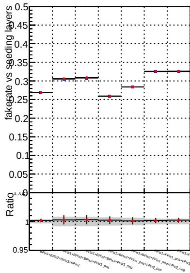
—●— DQM CKF TTbase —●— DQM CKF TT_retrainOldFiles125_v2_prelimWPM_epoch2
