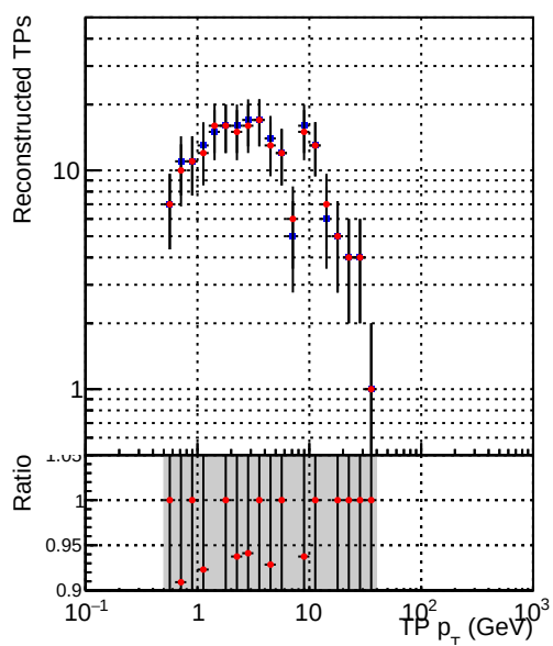
DQM_CKF_TTbase DQM_CKF_TT_retrainOldFiles125_v2_prelimWPM_epoch2
