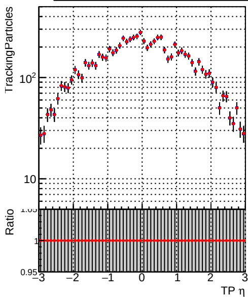
DQM_CKF_TTbase DQM_CKF_TT_retrainOldFiles125_v2_prelimWPM_epoch2
