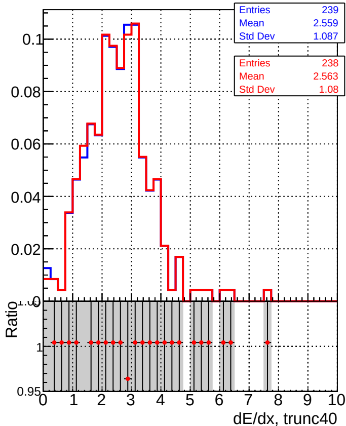
DQM_CKF_TTbase DQM_CKF_TT_retrainOldFiles125_v2_prelimWPM_epoch2
