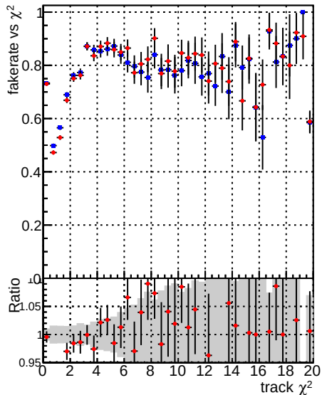
Fake rate vs. —●— DQM CKF TTbase —●— DQM CKF TT_retrainOldFiles125_v2_prelimWPM_epoch2
