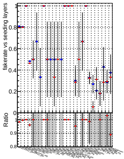
Fake rate vs. —●— DQM CKF TTbase —●— DQM CKF TT_retrainOldFiles125_v2_prelimWPM_epoch2
