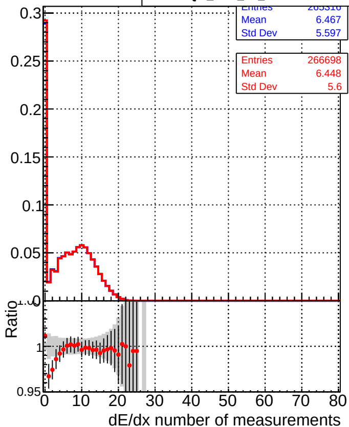
■ DQM_CKF_TTbase —●— DQM_CKF_TT_retrainOldFiles125_v2_prelimWPM_epoch2
