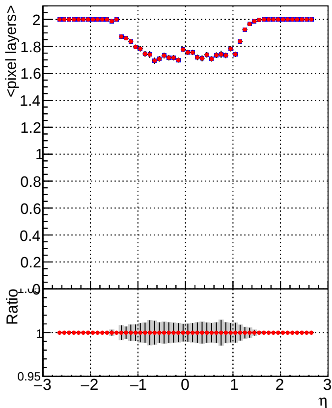
■ DQM_CKF_TTbase ■ DQM_CKF_TT_retrainOldFiles125_v2_prelimWPM_epoch1
