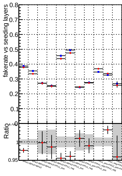
—●— DQM CKF TTbase —●— DQM CKF TT_retrainOldFiles125_v2_prelimWPM_epoch1
