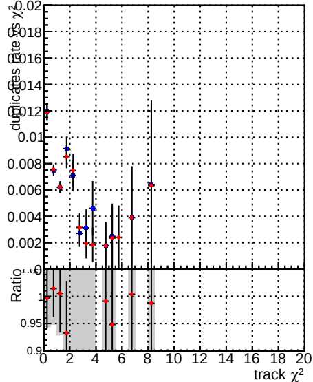
—●— DQM CKF TTbase —●— DQM CKF TT_retrainOldFiles125_v2_prelimWPM_epoch1
