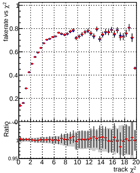
Fake rate vs. \chi^2 Legend: —•— DQM CKF TTbase —•— DQM CKF TT_retrainOldFiles125_v2_prelimWPM_epoch1
