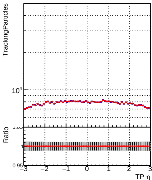
■ DQM_CKF_TTbase ■ DQM_CKF_TT_retrainOldFiles125_v2_prelimWPM_epoch1
