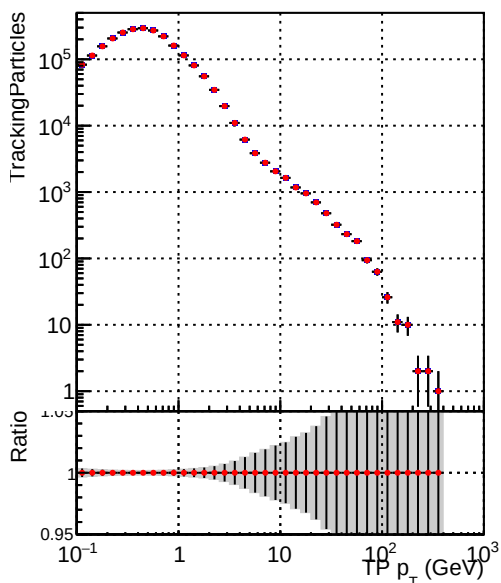
■ DQM_CKF_TTbase ■ DQM_CKF_TT_retrainOldFiles125_v2_prelimWPM_epoch1
