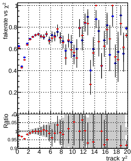
Fake rate vs. —•— DQM CKF TTbase —•— DQM CKF TT_retrainOldFiles125_v2_prelimWPM_epoch1
