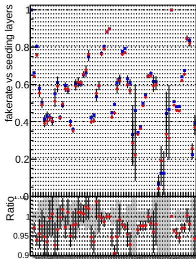
Fake rate vs. —•— DQM CKF TTbase —•— DQM CKF TT_retrainOldFiles125_v2_prelimWPM_epoch1
