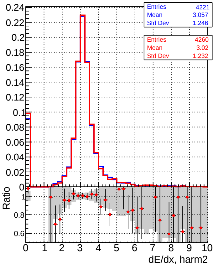
DQM_CKF_TTbase DQM_CKF_TT_retrainOldFiles125_v2_prelimWPM_epoch0
