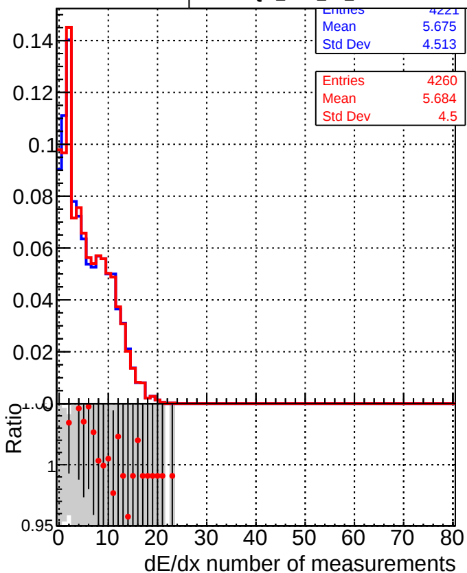
DQM_CKF_TTbase DQM_CKF_TT_retrainOldFiles125_v2_prelimWPM_epoch0
