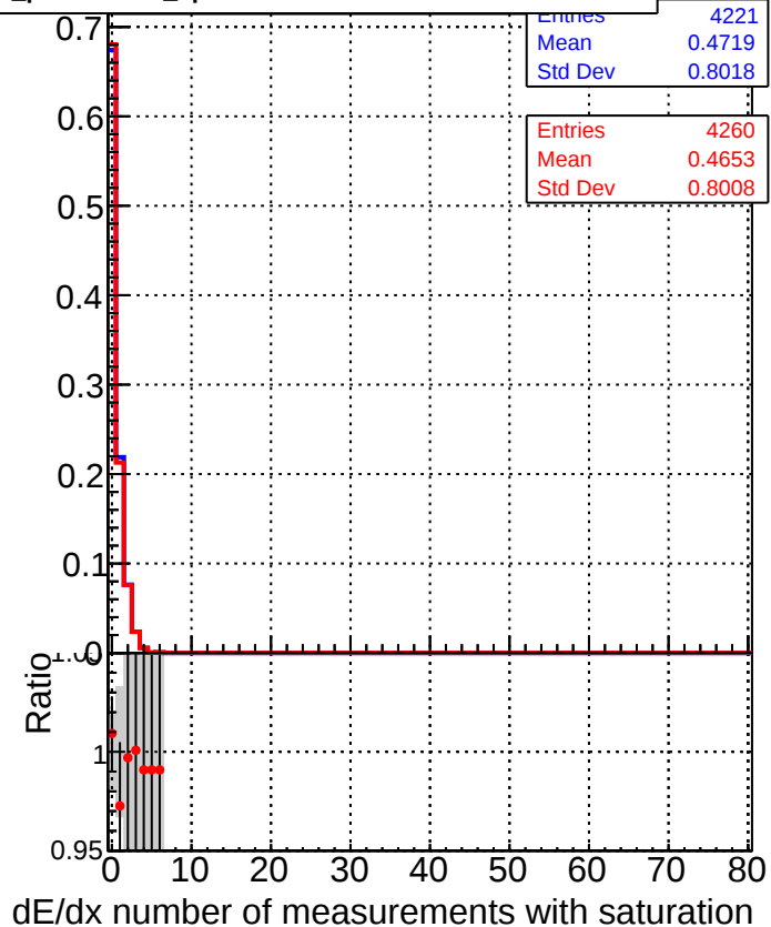
DQM_CKF_TTbase DQM_CKF_TT_retrainOldFiles125_v2_prelimWPM_epoch0
