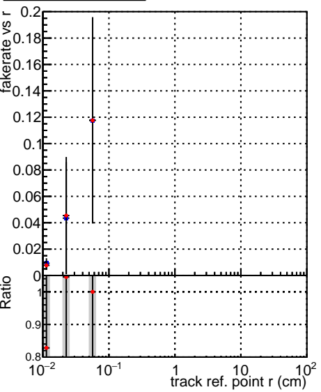
■ DQM_CKF_TTbase ● DQM_CKF_TT_retrainOldFiles125_v2_prelimWPM_epoch0
