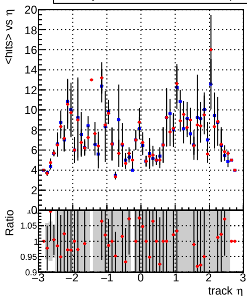
— DQM_CKF_TTbase — DQM_CKF_TT_retrainOldFiles125_v2_prelimWPM_epoch0
