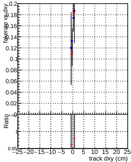
—●— DQM CKF TTbase —●— DQM CKF TT_retrainOldFiles125_v2_prelimWPM_epoch0
