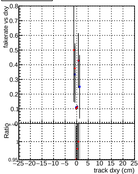
—●— DQM CKF TTbase —●— DQM CKF TT_retrainOldFiles125_v2_prelimWPM_epoch0
