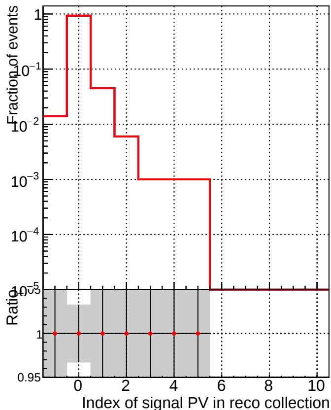
■ DQM_CKF_TTbase ● DQM_CKF_TT_retrainOldFiles125_v2_prelimWPM_epoch0
