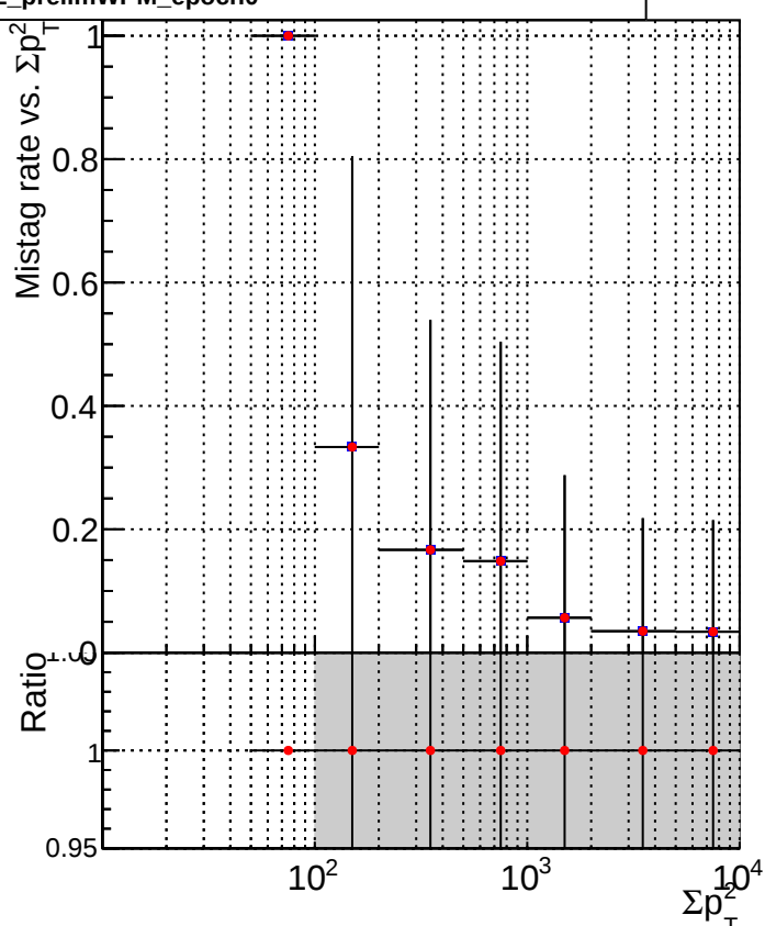
■ DQM_CKF_TTbase ● DQM_CKF_TT_retrainOldFiles125_v2_prelimWPM_epoch0
