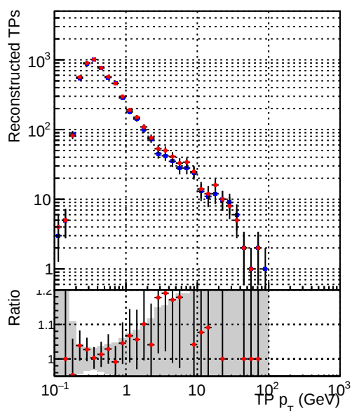
■ DQM_CKF_TTbase ■ DQM_CKF_TT_retrainOldFiles125_v2_prelimWPM_epoch0
