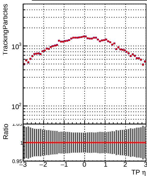
■ DQM_CKF_TTbase ■ DQM_CKF_TT_retrainOldFiles125_v2_prelimWPM_epoch0
