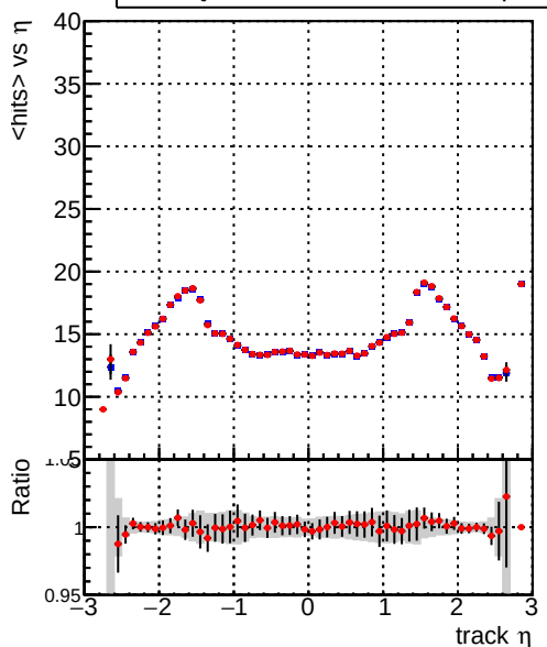
— DQM_CKF_TTbase — DQM_CKF_TT_retrainOldFiles125_v2_prelimWPM_epoch0
