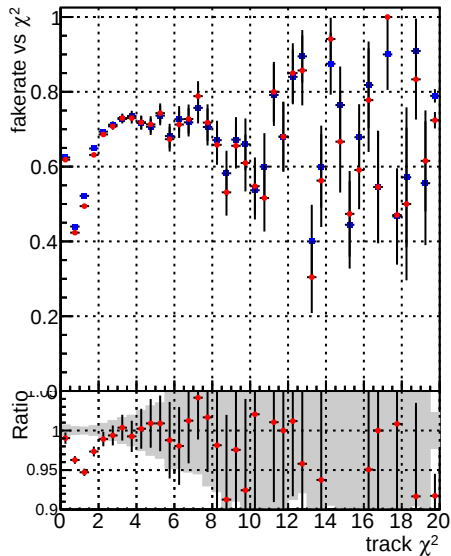
Fake rate vs. —•— DQM CKF TTbase —•— DQM CKF TT_retrainOldFiles125_v2_prelimWPM_epoch0
