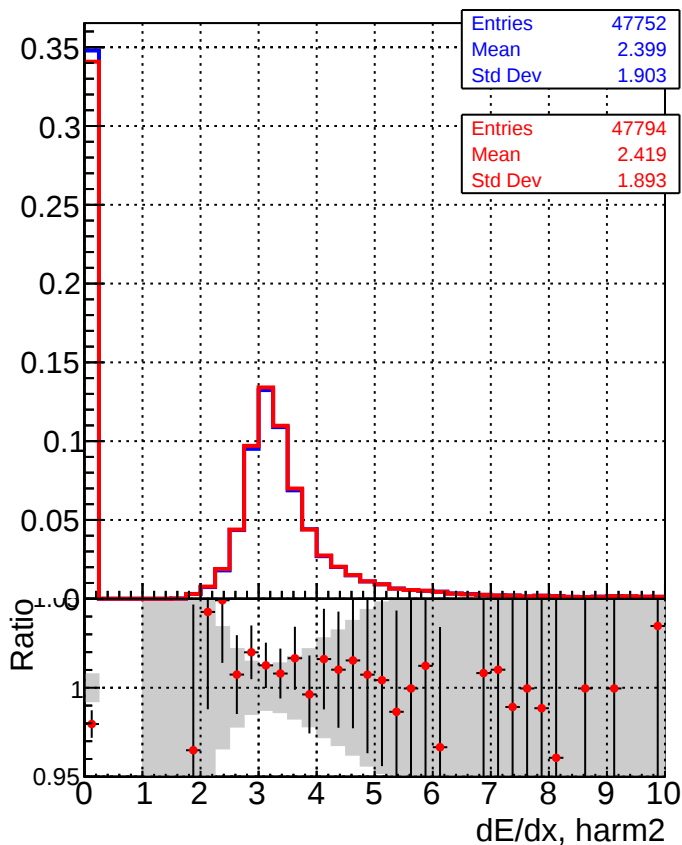
■ DQM_CKF_TTbase ● DQM_CKF_TT_retrainOldFiles125_v2_prelimWPM_epoch0
