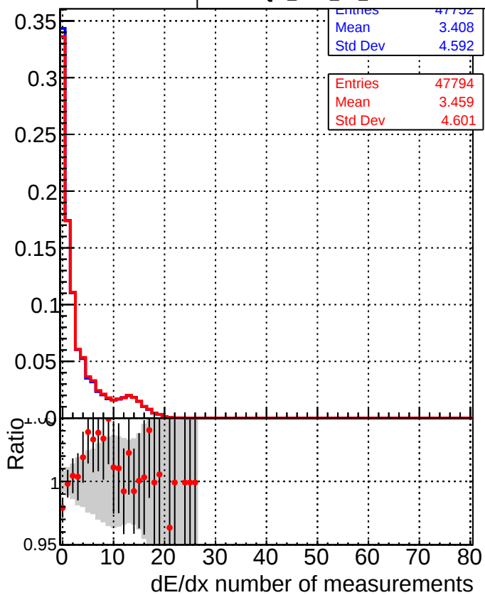
■ DQM_CKF_TTbase ● DQM_CKF_TT_retrainOldFiles125_v2_prelimWPM_epoch0
