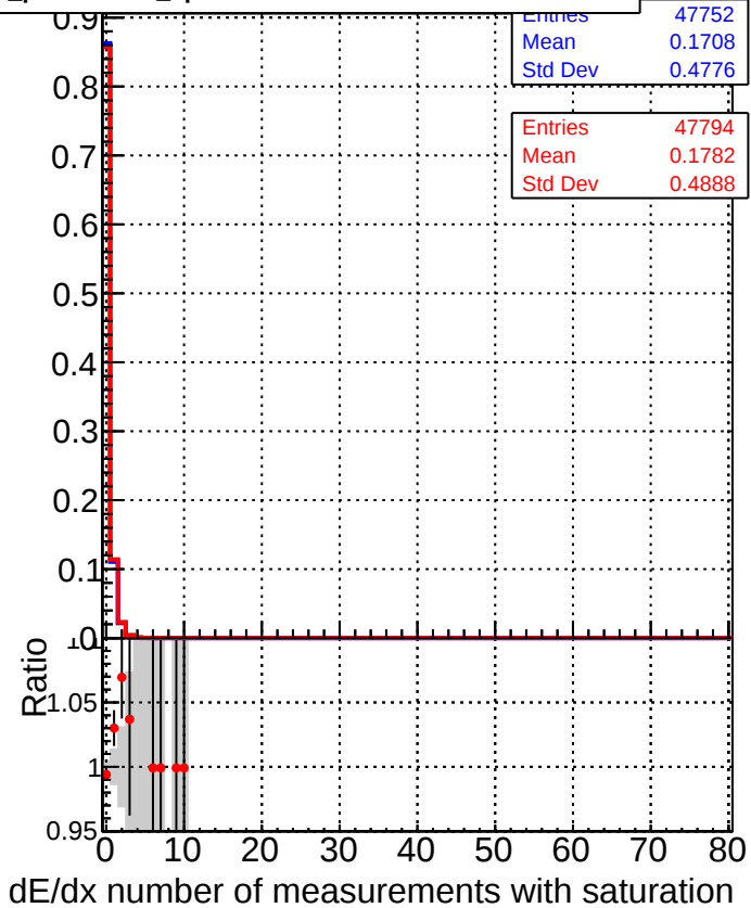
■ DQM_CKF_TTbase ● DQM_CKF_TT_retrainOldFiles125_v2_prelimWPM_epoch0
