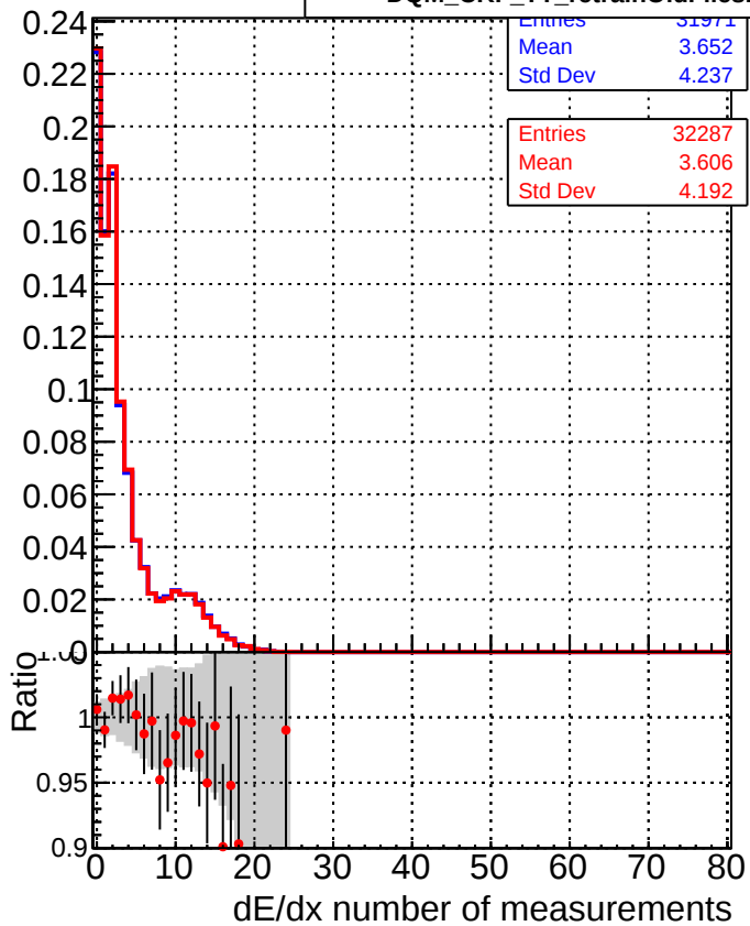
■ DQM_CKF_TTbase ● DQM_CKF_TT_retrainOldFiles125_v2_prelimWPM_epoch0
