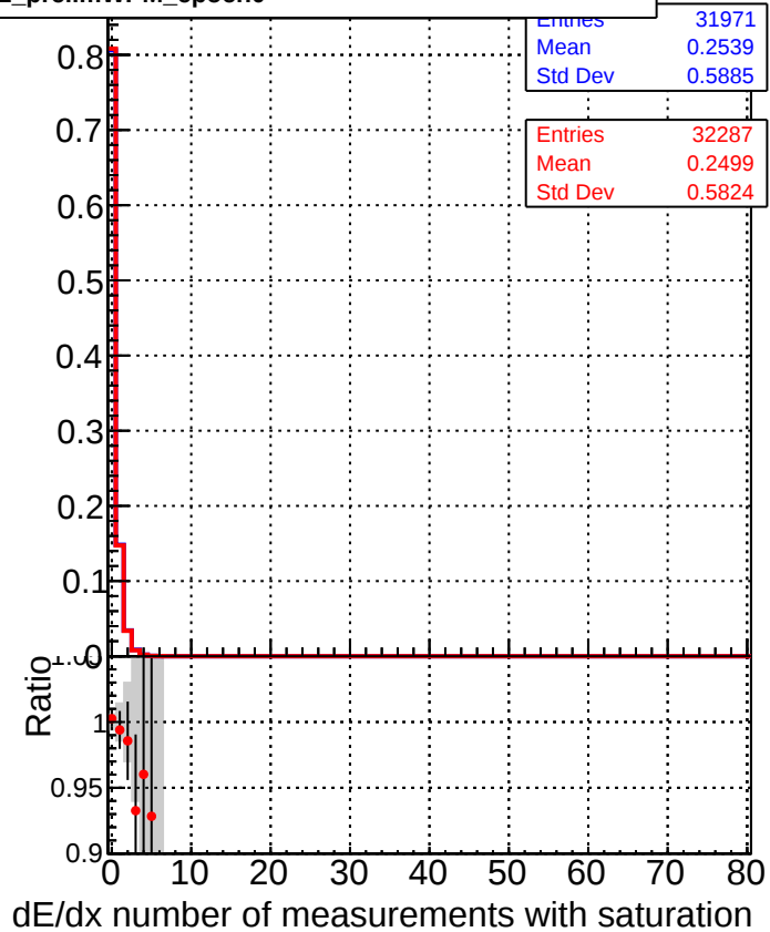
■ DQM_CKF_TTbase ● DQM_CKF_TT_retrainOldFiles125_v2_prelimWPM_epoch0
