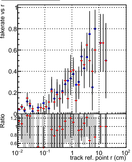
—●— DQM_CKF_TT_retrain —●— DQM_mkFit_TT_retrain
