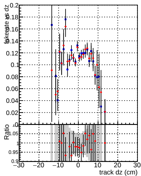
Fake rate vs dz — DQM_CKF_TT_retrain — DQM_mkFit_TT_retrain
