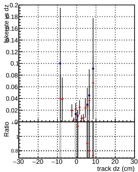
—●— DQM_CKF_TT_retrain —●— DQM_mkFit_TT_retrain
