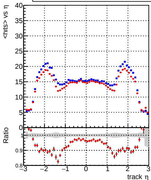
mean hits vs \eta — DQM_CKF_TT_retrain — DQM_mkFit_TT_retrain
