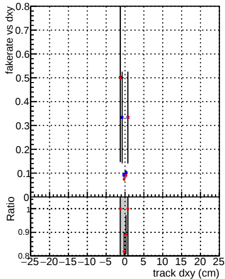
—•— DQM_CKF_TT_retrain —•— DQM_mkFit_TT_retrain
