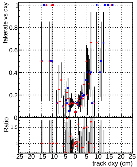
—■— DQM_CKF_TT_retrain —●— DQM_mkFit_TT_retrain
