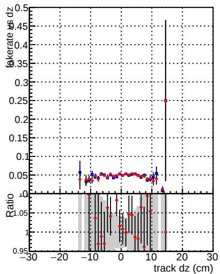
—■— DQM_CKF_TT_retrain —●— DQM_mkFit_TT_retrain
