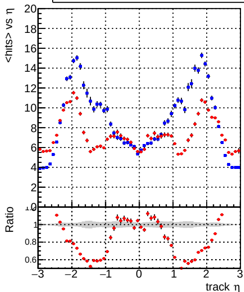
mean hits — DQM_CKF_TT_retrain — DQM_mkFit_TT_retrain
