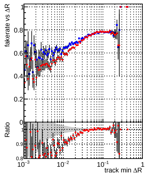
—•— DQM_CKF_TT_retrain —•— DQM_mkFit_TT_retrain
