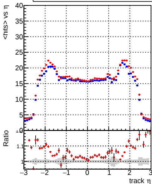
mean hits — DQM_CKF_TT_retrain — DQM_mkFit_TT_retrain
