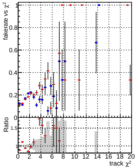
Fake rate vs. — DQM CKF TT_base — DQM mkFit TT_base
