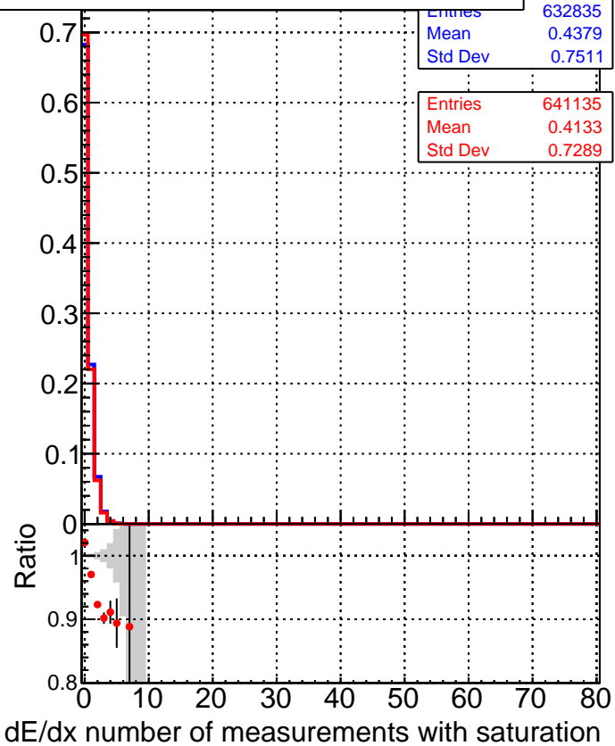
■ DQM_CKF_TT_base ● DQM_mkFit_TT_base
