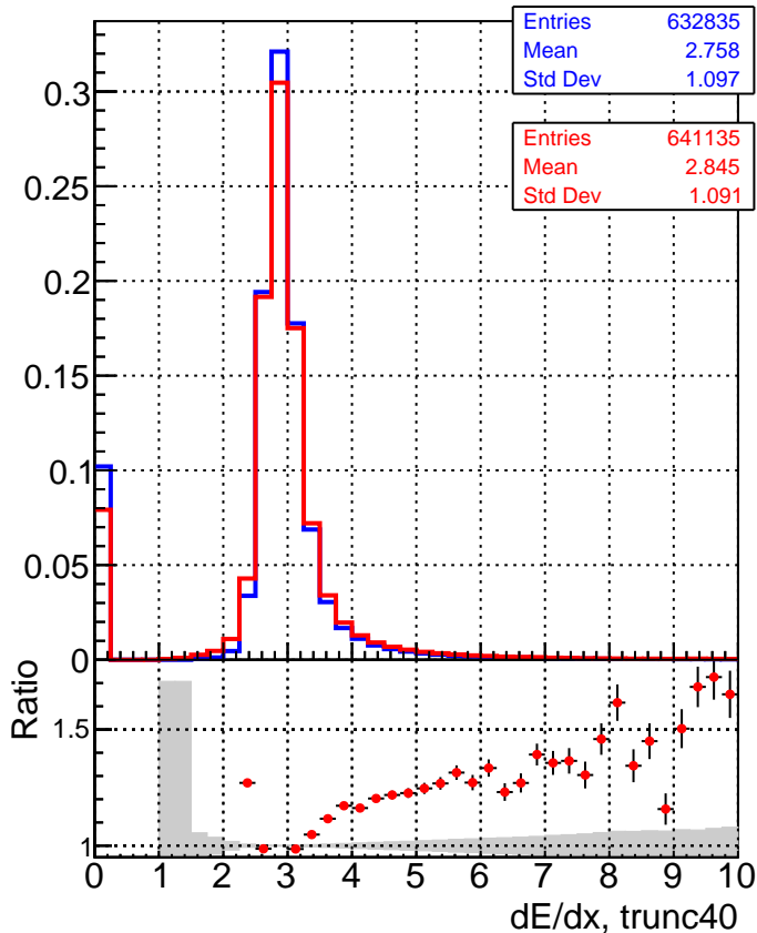
■ DQM_CKF_TT_base ● DQM_mkFit_TT_base
