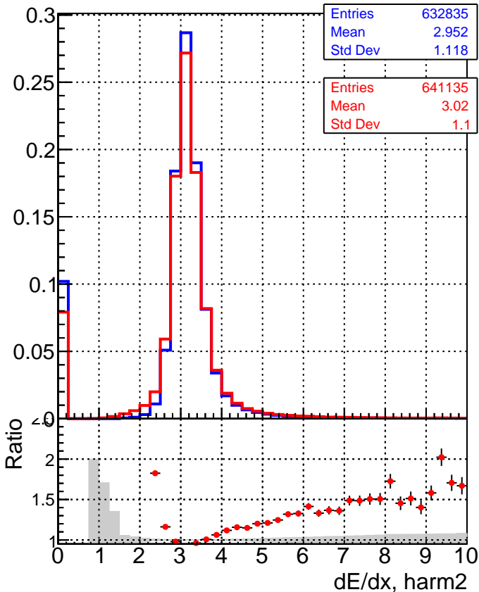
■ DQM_CKF_TT_base ● DQM_mkFit_TT_base
