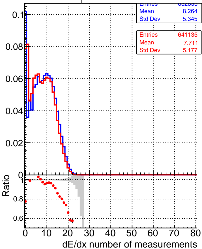
■ DQM_CKF_TT_base ● DQM_mkFit_TT_base
