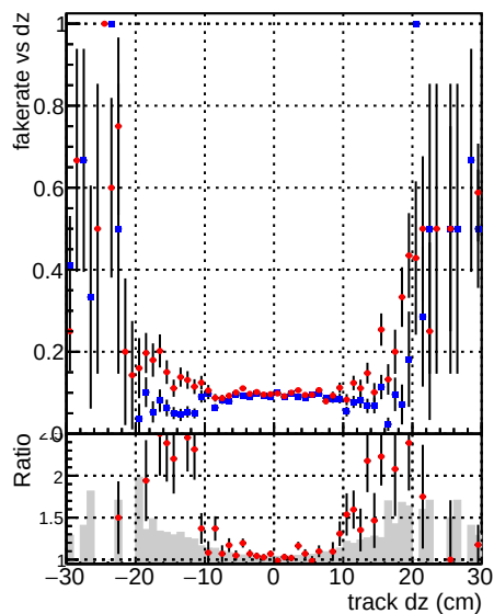
Fake rate vs dz —■— DQM CKF TT_base —●— DQM mkFit TT_base
