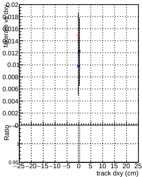
—●— DQM CKF TT_base —●— DQM mkFit TT_base
