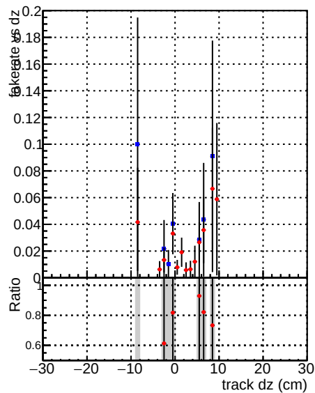
—●— DQM CKF TT_base —●— DQM mkFit TT_base
