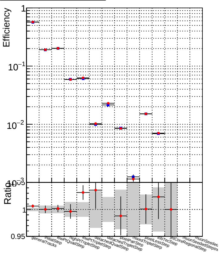
DQM_mkFit_TT_base DQM_mkFit_TT_retrain
