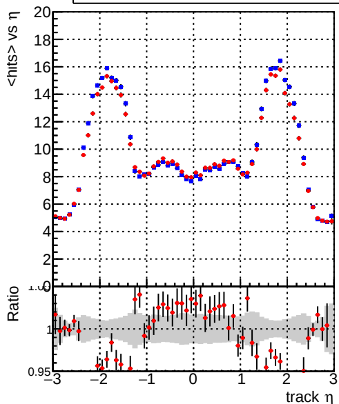
DQM_mkFit_TT_base mean hit DQM_mkFit_TT_retrain
