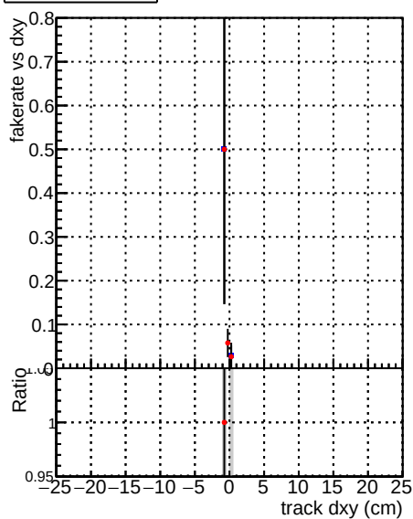
—•— DQM_mkFit_TT_base —•— DQM_mkFit_TT_retrain
