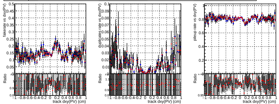
Fake rate vs d DQM_mkFit_TT_base DQM_mkFit_TT_retrain
