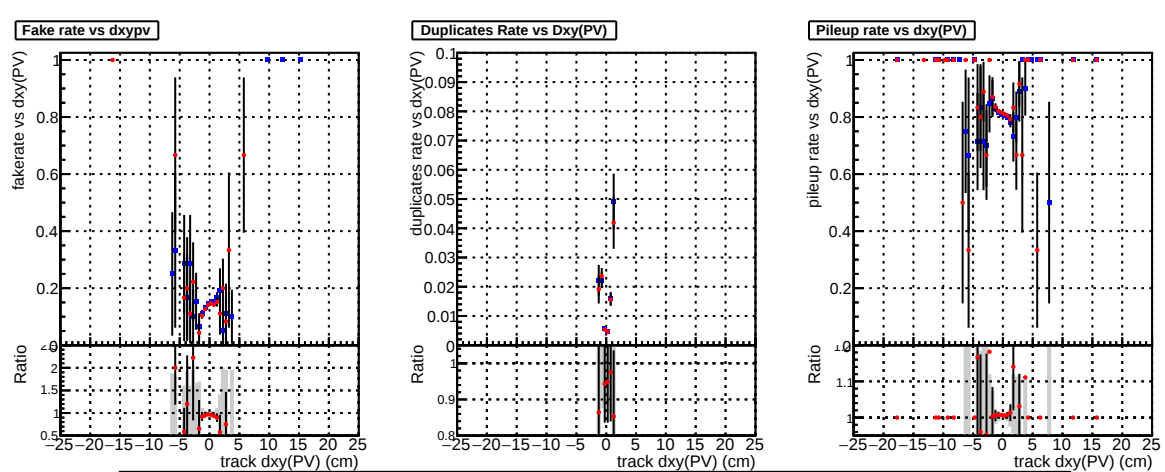
Fake rate vs d DQM_mkFit_TT_base DQM_mkFit_TT_retrain
