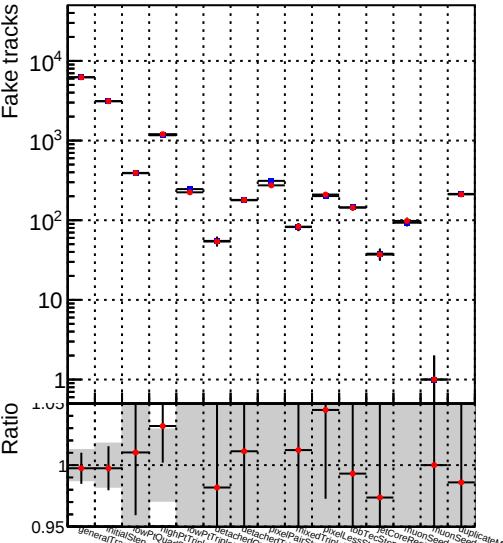
Number —●— DQM_mkFit_TT_retrain
